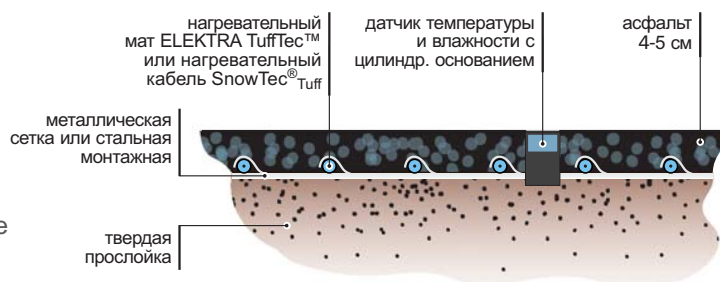
Поперечное сечение дороги из асфальта (установка непосредственно в асфальт)
