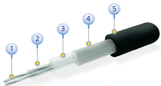
Конструкция нагревательного кабеля ELEKTRA TuffTec™
