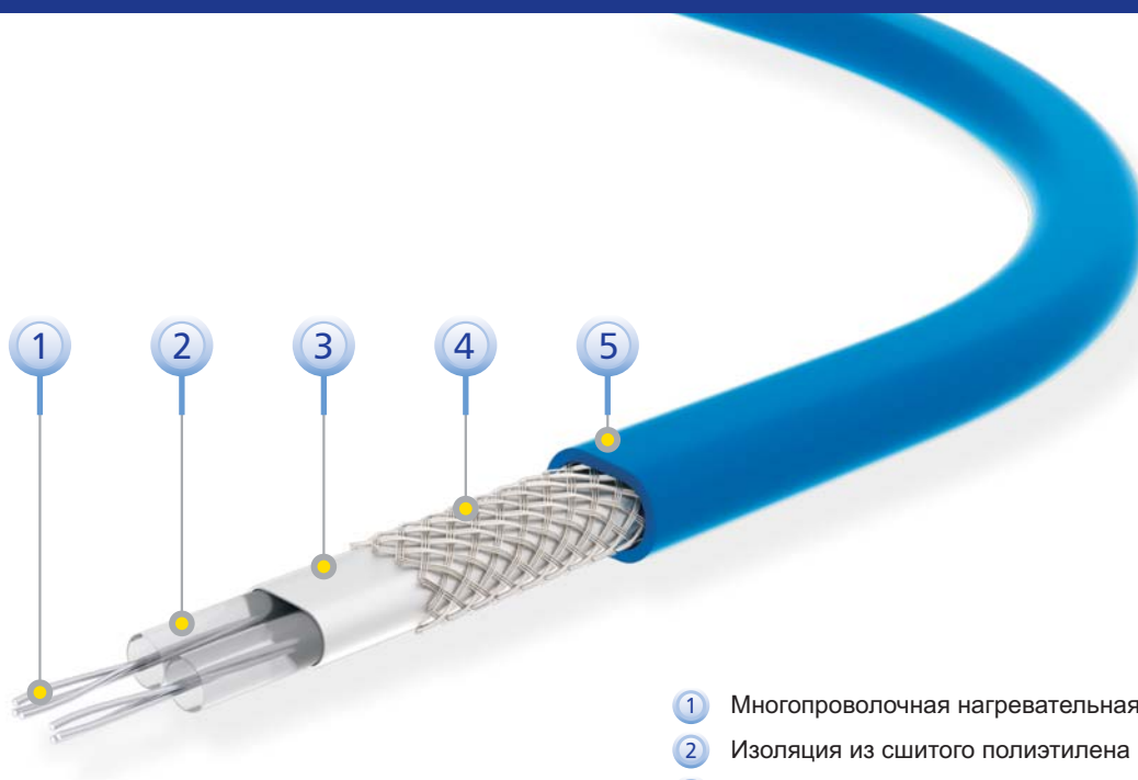
Конструкция нагревательного кабеля ELEKTRA VCD
